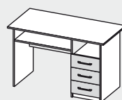
Стол письменный 1100x750x600
