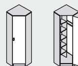
Шкаф угл. 908x2200x908
