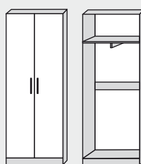
Шкаф 2-ств. 556x2200x374
