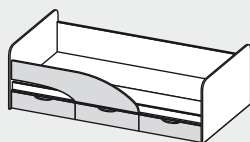
Кровать - 3 лев./прав. 1942x700x862
