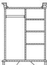
Шкаф П02Б L1470xB650xH2110
