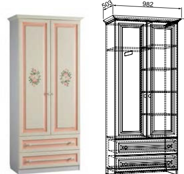
12 Шкаф 2-створчатый «Алиса» → | 7 | ↑ 982|503|2148
