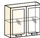
13 Шкаф навесной (2 двери рамочные) → | 7 | ↑ 800|318|720
