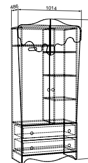
3 Шкаф 2-створчатый с ящиками «Пряничный домик» → | 7 | ↑ 1014|486|2135
