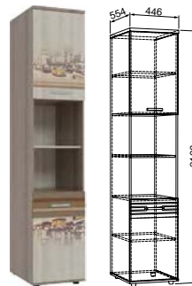
9 Шкаф комбинированный «Манхэттен» → | 7 | ↑ 446|554|2198
