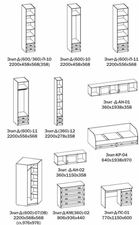
Элит-Д-КР-04-К 640x1938x970 / Элит-Д-КМ(360)-02-К 806x936x440 / Элит-Д-(360)-П-10-Л 2200x458x358 / Элит-Д-АН-02 360x1150x358 Элит-Д-ПС-01-К 770x1150x600 / Элит-Д-(360)-12-Л 2200x278x358
